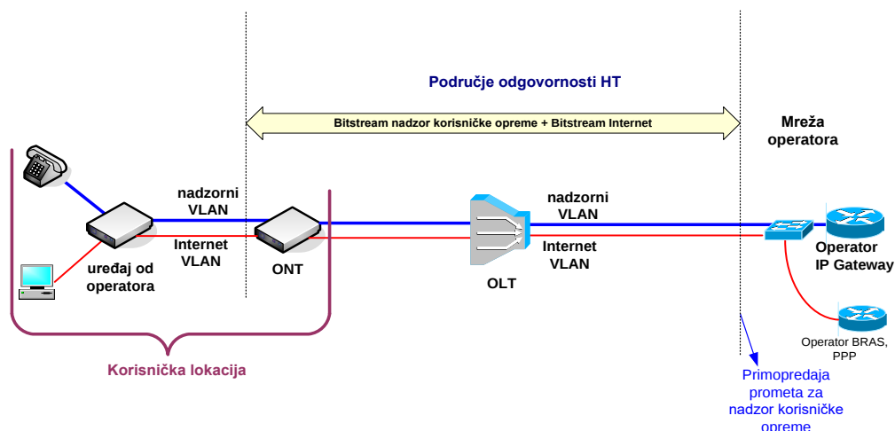
Slika 28. Veleprodajni širokopojasni pristup za pružanje usluge nadzora korisničke opreme preko FTTH pristupa (GPON) na OLT razini
