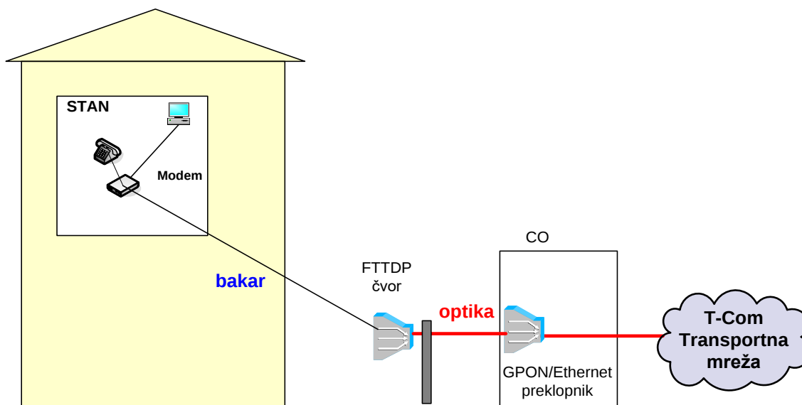
Slika 36. Način realizacije FTTPD koncepta sa VDSL17a tehnologijom u pristupnoj mreži
